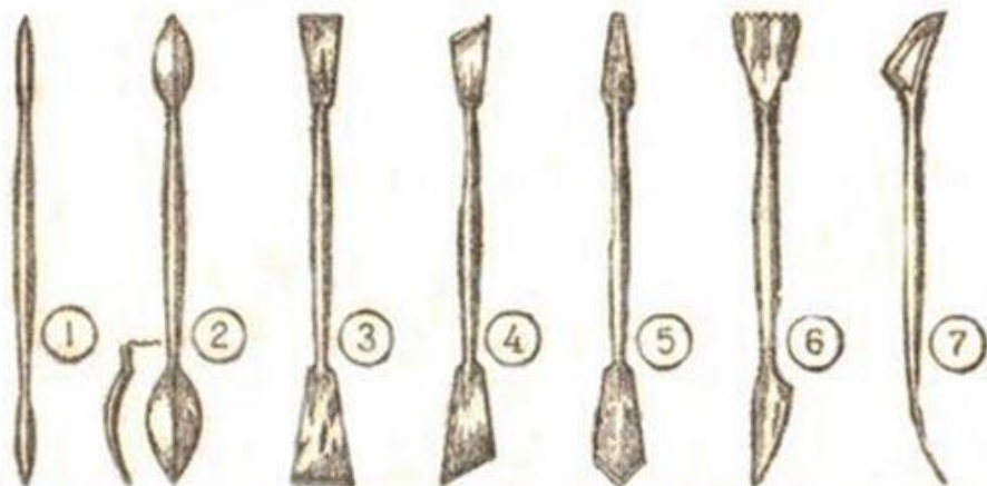
1 ЦАРАПКА СТАЛЬНАЯ 2 ЛОЖКА 3 ДОЛОТО ПРЯМОЕ 4 ДОЛОТО КОСОЕ 5 ДОЛОТО КОПЬЕВИДНОЕ 6 ЗУБЧАТКА И КОСАРЬ 7 СТЯКА СТАЛЬНАЯ ИНСТРУМЕНТЫ ДЛЯ РУЧНОГО ВЫРЕЗАНИЯ СГРАФФИТО
